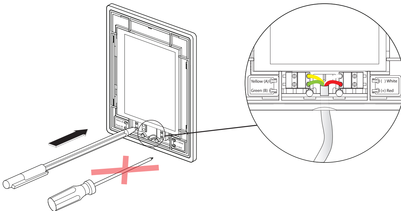
Obr. 17 Káblové pripojenie k ovládaciemu panelu
