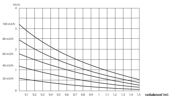
RONDO 100/125 rýchlosť, m/s
