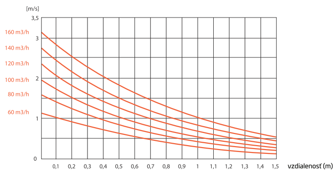
RONDO 160 rýchlosť, m/s
